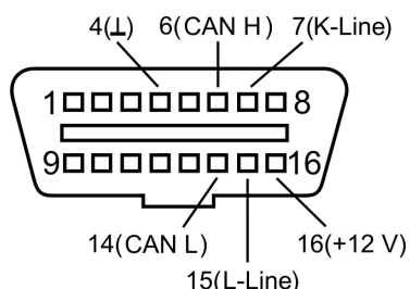
Рис. 2. Диагностический разъем OBD-II, используемый в автомобилях VAG с 1994 г.
