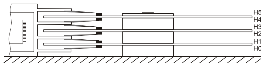
Рис.5.1.3. Расположение магнитных поверхностей WDAC31200.
