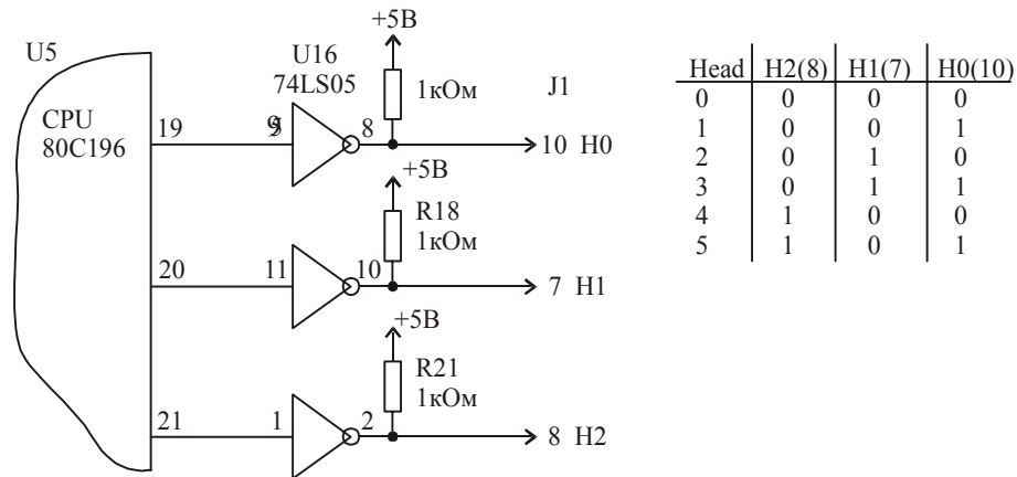
Рис. 5.2.4. Схема выбора магнитных головок накопителей семейства WDAC31000.
