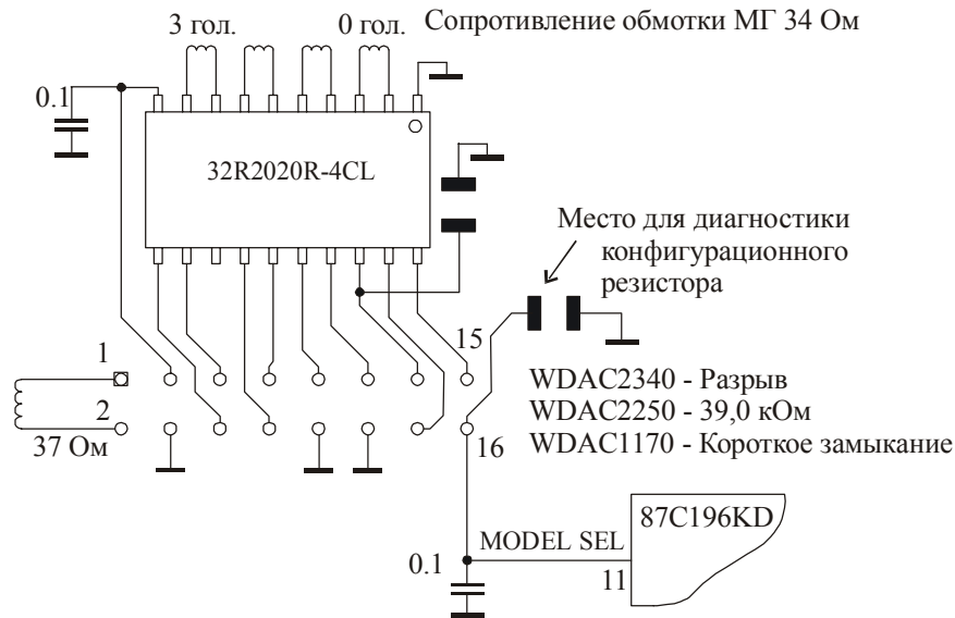
Рис. 5.5.4. Переконфигурация HDD семейства WDAC2340.
