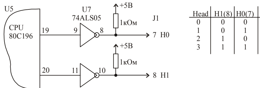
Рис. 5.3.4. Схема выбора магнитных головок накопителей семейства WDAC2540.
