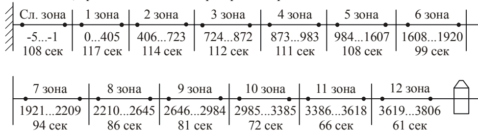
Рис. 5.2.1. Структура дискового пространства накопителей семейства WDAC31000.
