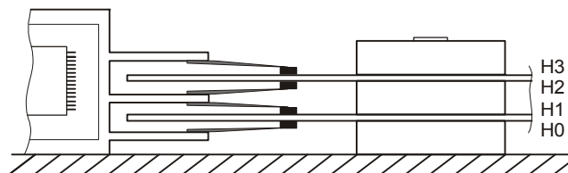
Рис. 5.3.2. Расположение магнитных поверхностей WDAC2540. (WDAC1270 имеет только 1 диск (0,1 поверхность)).
