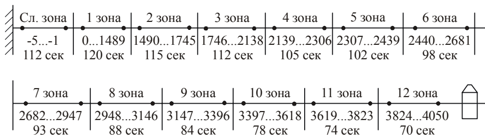
Рис.5.1.2. Структура дискового пространства накопителей семейства WDAC31200.
