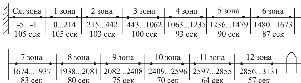
Рис.5.3.2. Структура дискового пространства накопителей семейства WDAC2540
