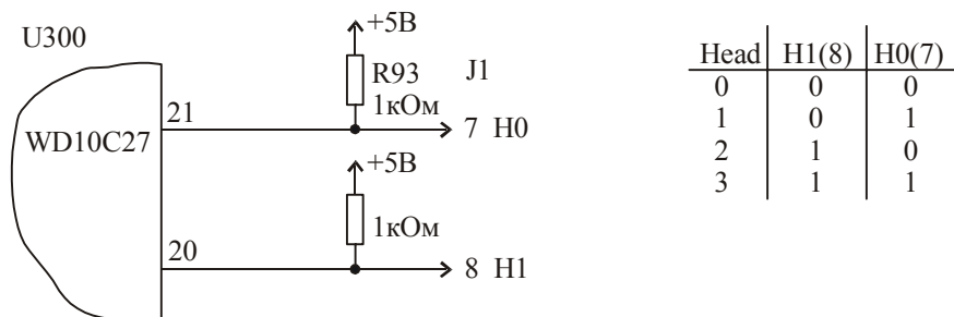
Рис. 5.4.5. Схема выбора магнитных головок накопителей семейства WDAC2420.
