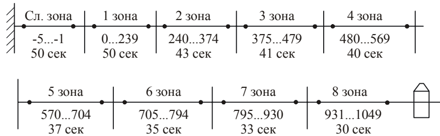
Рис. 5.4.2 Структура дискового пространства накопителей семейства WDC CU140
