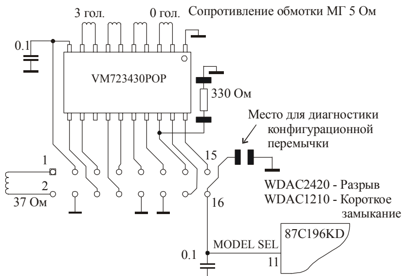
Рис. 5.4.4. Переконфигурация HDD семейства WDAC2420.
