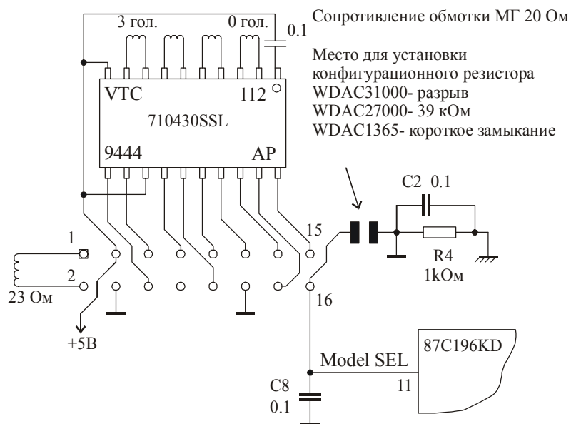
Рис. 5.2.3. Переконфигурация HDD семейства WDAC31000.
