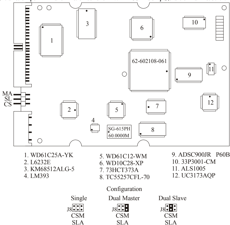
Рис. 5.1.1. Внешний вид платы электроники накопителей семейства WDAC31200
