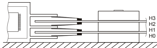
Рис. 5.4.3. Расположение магнитных поверхностей WDAC2420. (WDAC1210 имеет только 1 диск (0,1 поверхность)).
