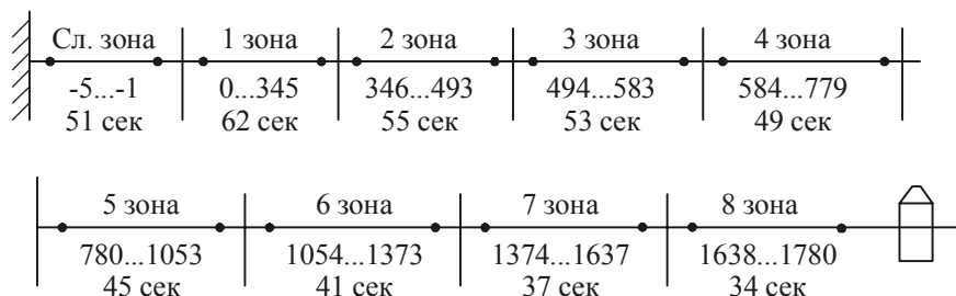
Рис. 5.6.1. Структура дискового пространства накопителей семейства WD AL2170.
