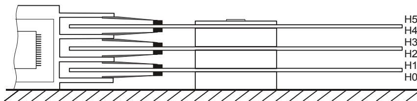
Рис. 5.2.2. Расположение магнитных поверхностей WDAC31000. (WDAC2700 имеет 2-а диска (0,1,2,3 поверхности, WDAC1365 имеет только 1 диск (0,1 поверхности ).
