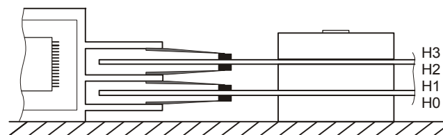
Рис. 5.5.3. Расположение магнитных поверхностей WDAC2340. (WDAC1170 имеет только 1 диск (0,1 поверхность), WDAC2250 имеет 2-а диска (0,1,2 поверхности).
