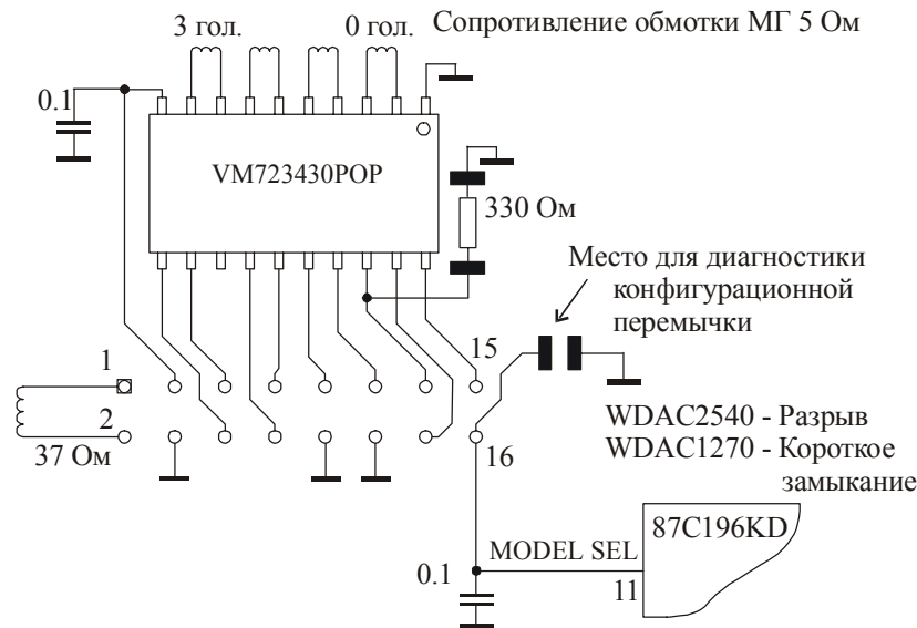
Рис. 5.3.3. Переконфигурация HDD семейства WDAC2540.
