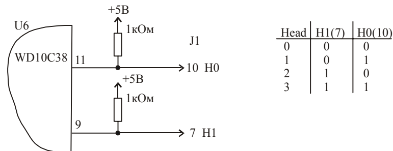
Рис. 5.5.5. Схема выбора магнитных головок накопителей семейства WDAC2340.
