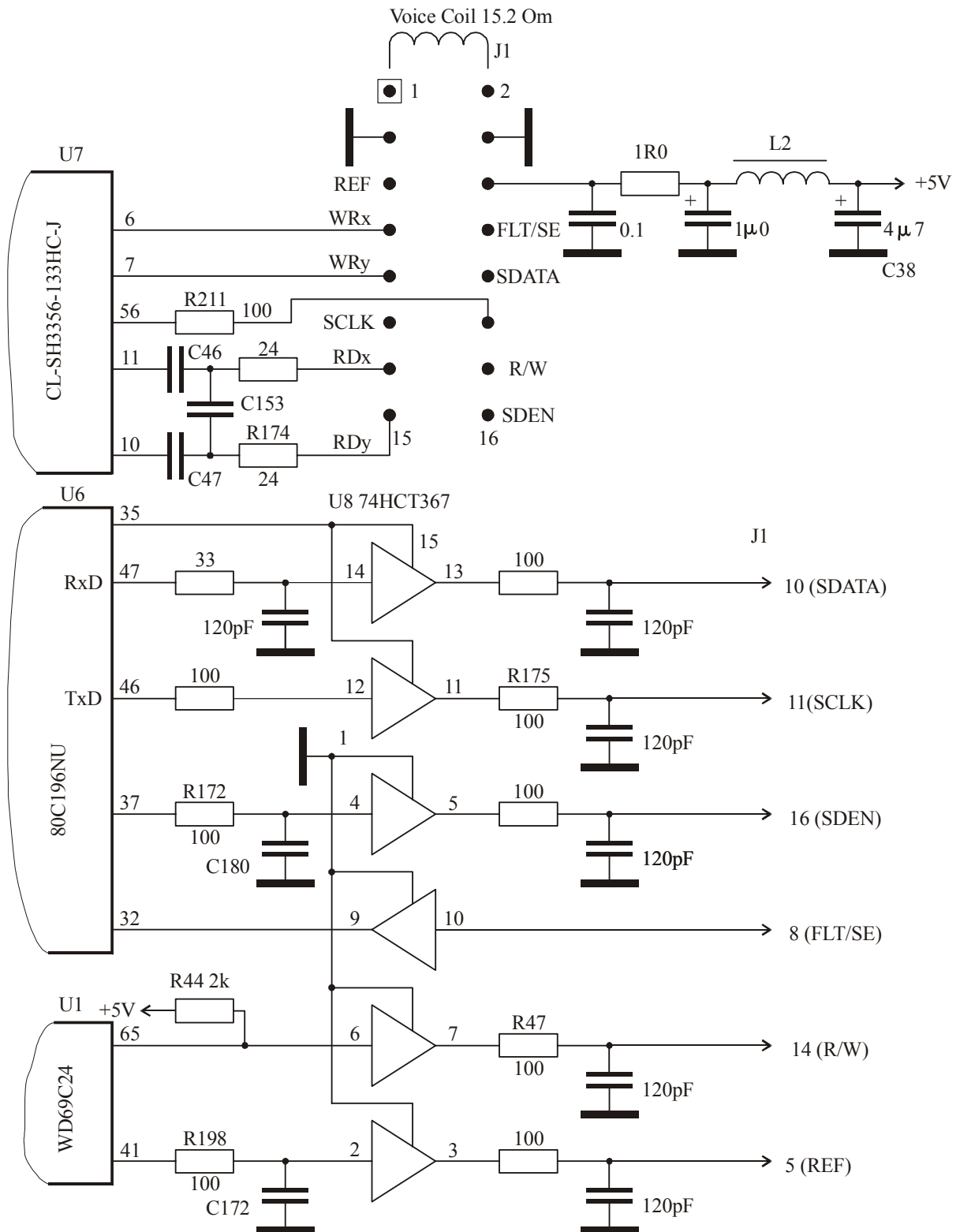
Рис. 5.3.7. Разъем J1 семейства WDAC36400.
