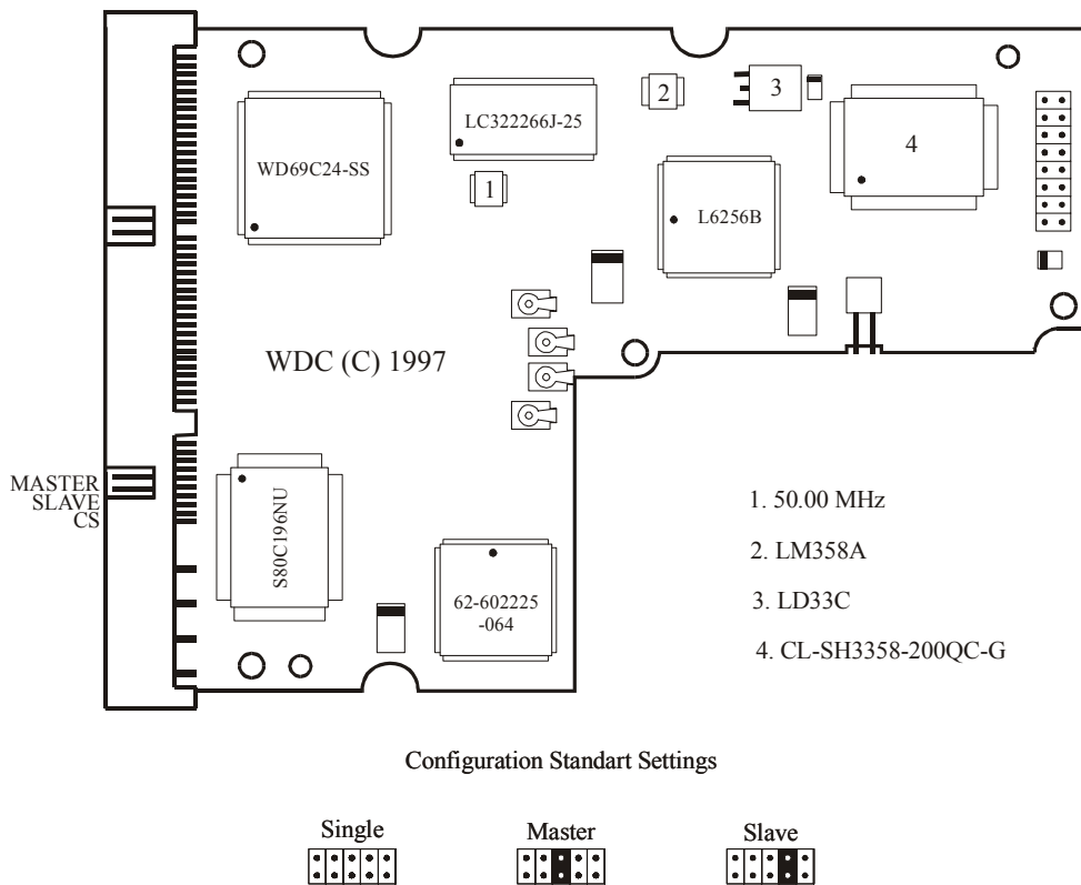
Рис.5.3.3. Внешний вид платы электроники накопителей семейства WDAC38400.
