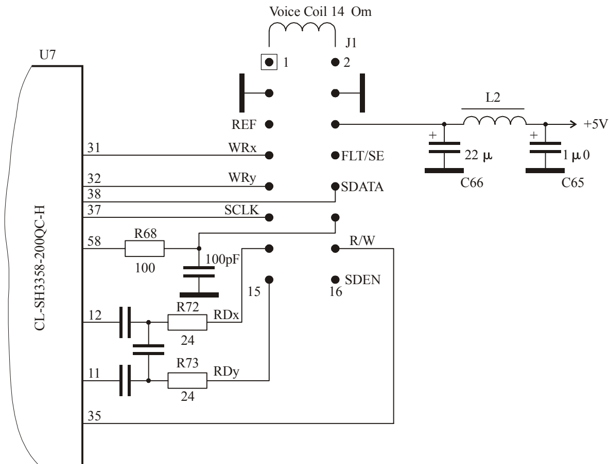
Рис. 5.3.8. Разъем J1 семейства WDAC310100.
