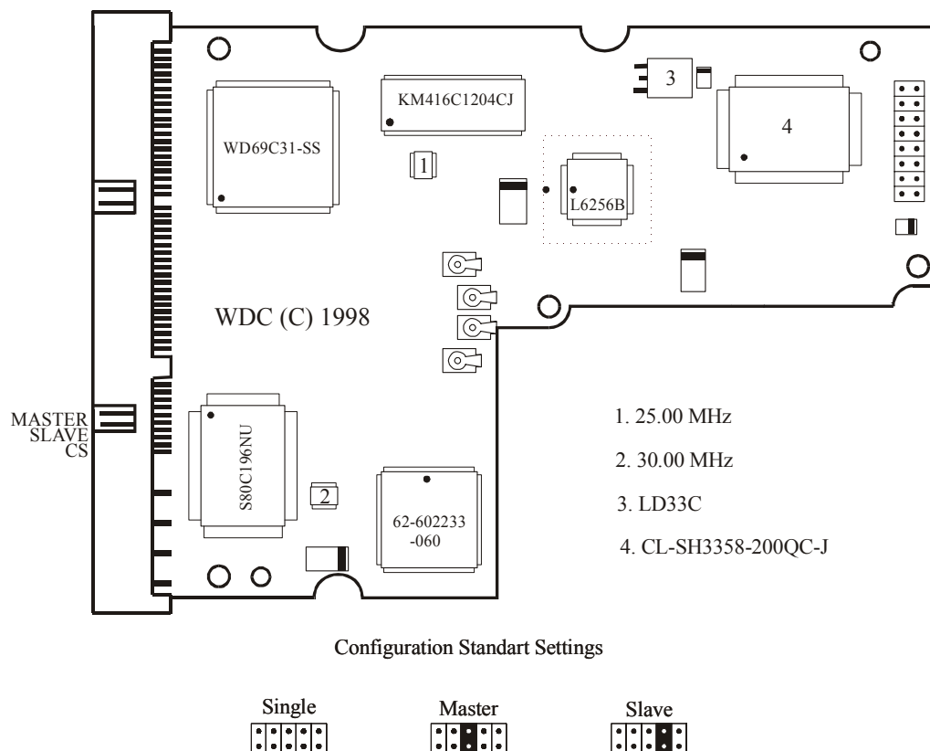
Рис.5.3.1. Внешний вид платы электроники накопителей семейства WDAC313000.
