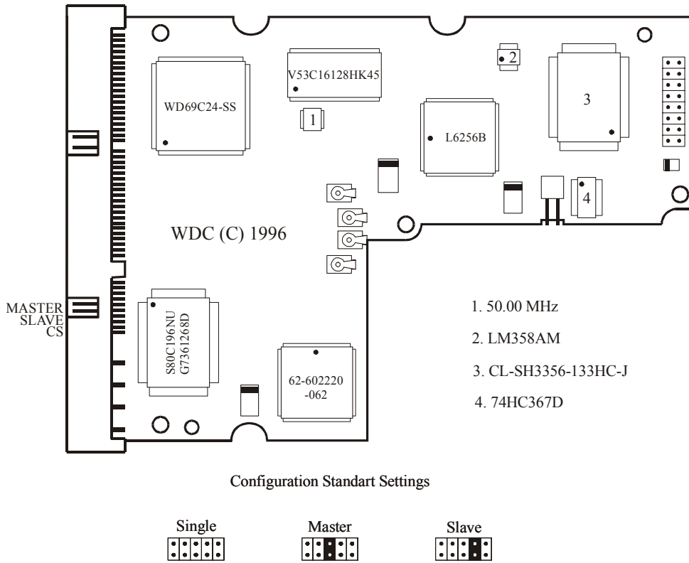
Рис.5.3.4. Внешний вид платы электроники накопителей семейства WDAC36400.
